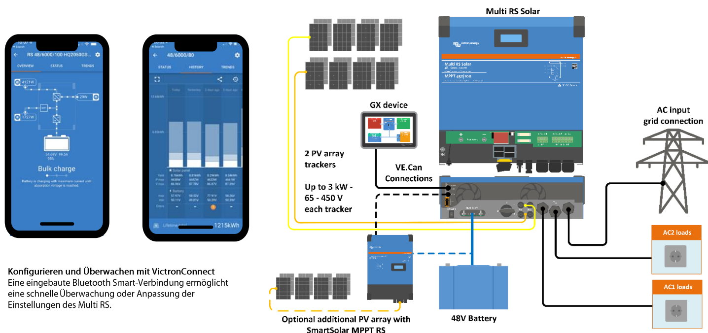
Blockdiagramm von Multi RS Solar
