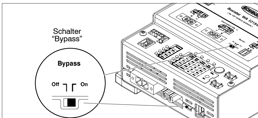
Bild 13 Schiebeschalter "Bypass"
