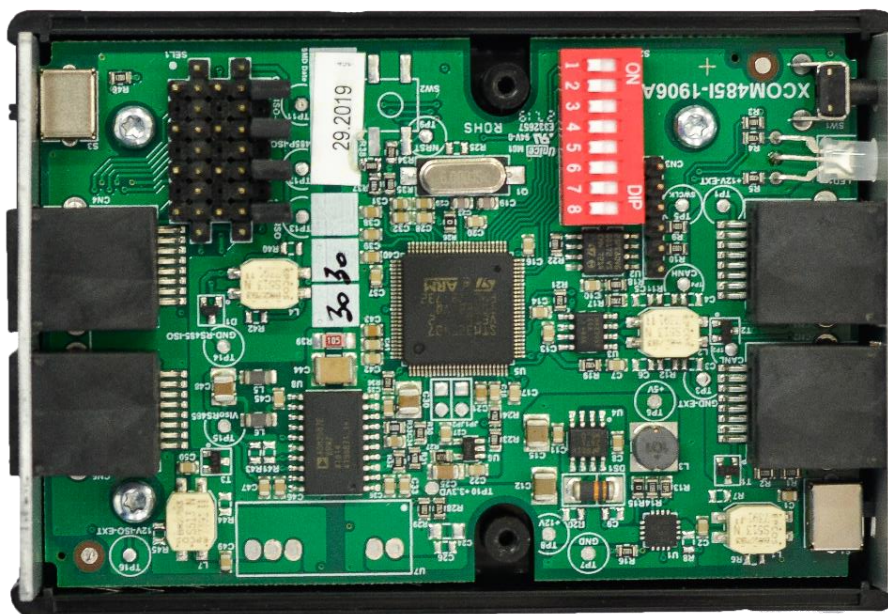
Abbildung 1: Leiterplatte im Xcom-485.
